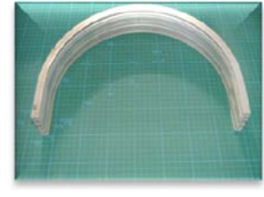
アルミ合金60系異型材 E65 × t3.0 × R170 Aluminum alloy(60 series)
